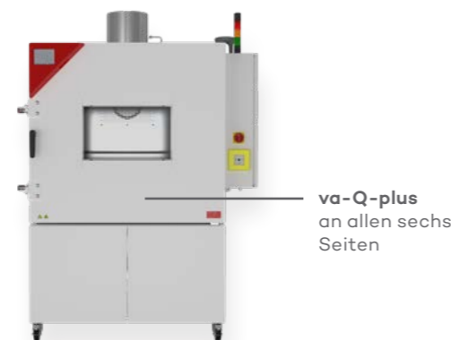
BINDER Batterie-Prüfschrank für Temperatur- und Sicherheitstests im Labor
